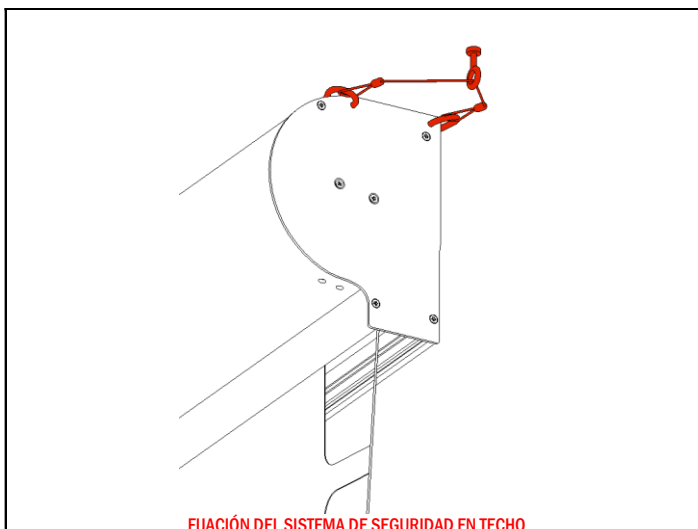
FIJACIÓN DEL SISTEMA DE SEGURIDAD EN TECHO
