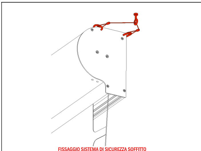
FISSAGGIO SISTEMA DI SICUREZZA SOFFITTO
