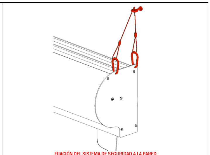
FIJACIÓN DEL SISTEMA DE SEGURIDAD A LA PARED
