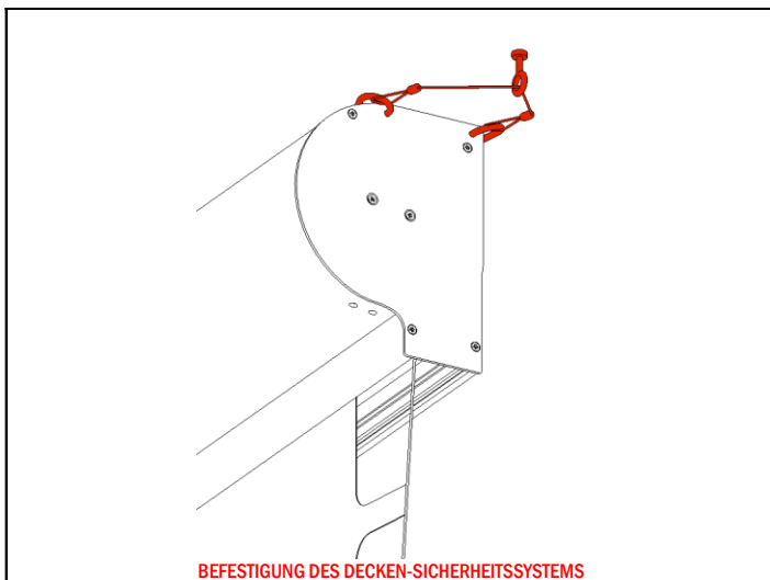
BEFESTIGUNG DES DECKEN-SICHERHEITSSYSTEMS
