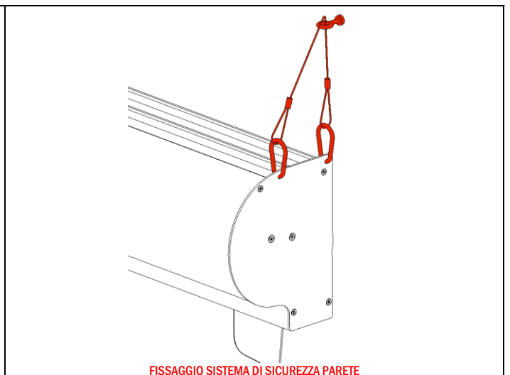
FISSAGGIO SISTEMA DI SICUREZZA PARETE
