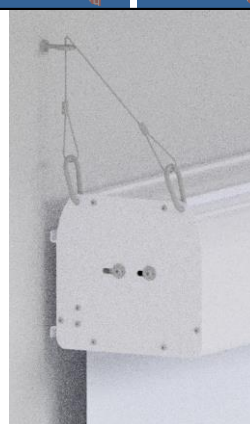
FISSAGGIO SISTEMA DI SICUREZZA
